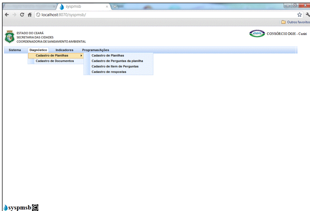
Figura 3.1. Menu Diagnóstico
