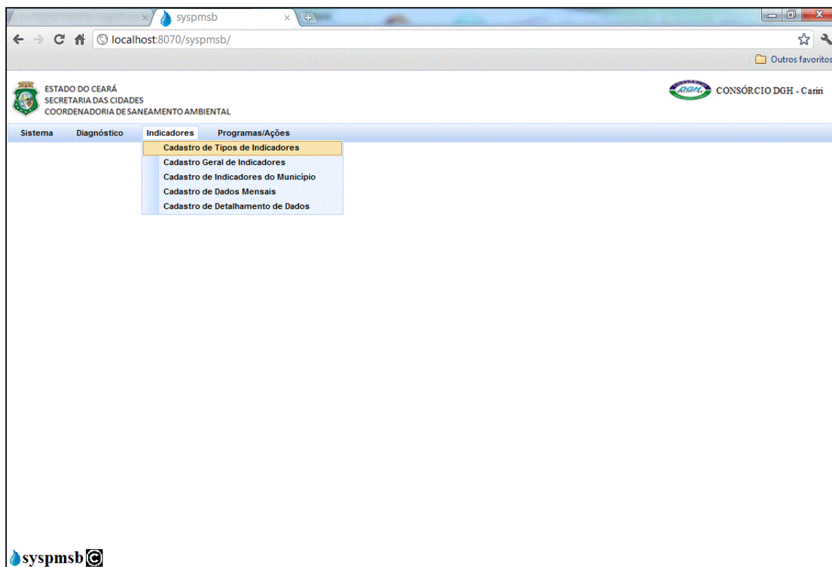
Figura 3.1. Menu Indicadores
